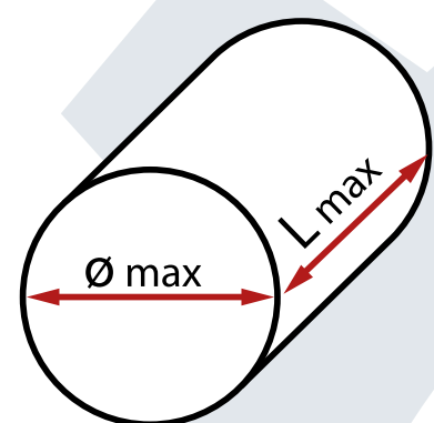
TORNITURA ASSIALE con utensili motorizzati Ø 500 mm L 1000 mm
