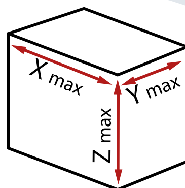
FRESATURA X 2000 mm Y 670 mm Z 600 mm
